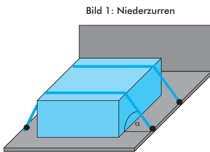
große Vorspannkraften
